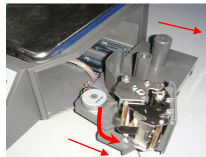
(2) Σύρατε προς τα έξω τον εκτυπωτή και ανοίξτε την περιστρεφόμενη μονάδα εκτύπωσης
